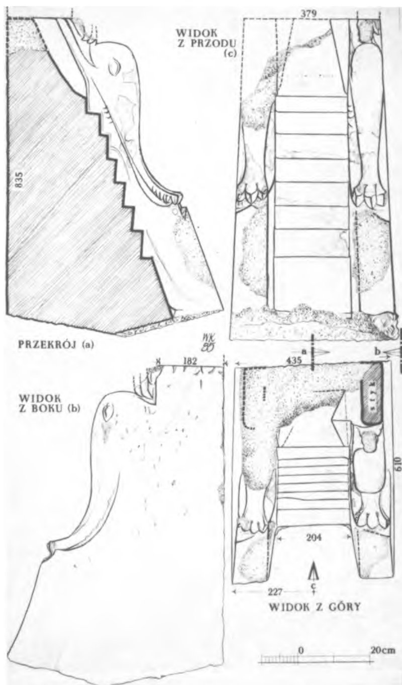
Ryc. 3. Schody wodne (por. ryc. 1). Rys. W. Klinger
