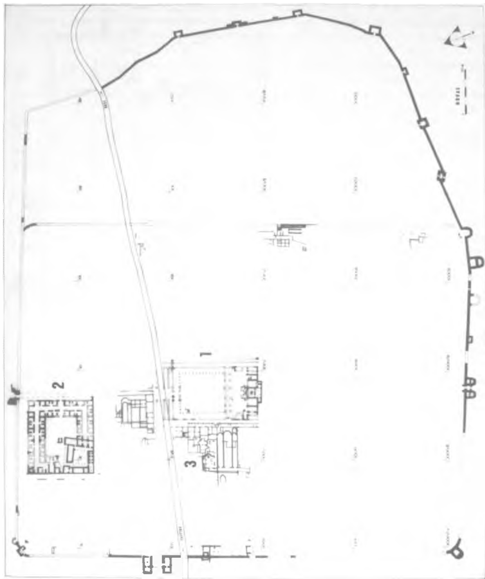
Ryc. 1. Novae. Plan ogólny. 1 – principia , 2 – basylia i rezydencja biskupia. Oprac. A. Biernacki, T. Samowski
