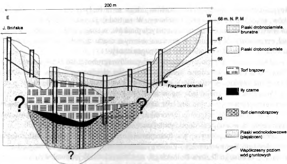
Ryc. 4. Błazejewo, gm. Kórnik, woj. wielkopolskie, stan. 4. Przekrój geologiczny przez zachodnią terasę Jeziora Bnińskiego (por. ryc. 1B). Rys. J. Jasiewicz
