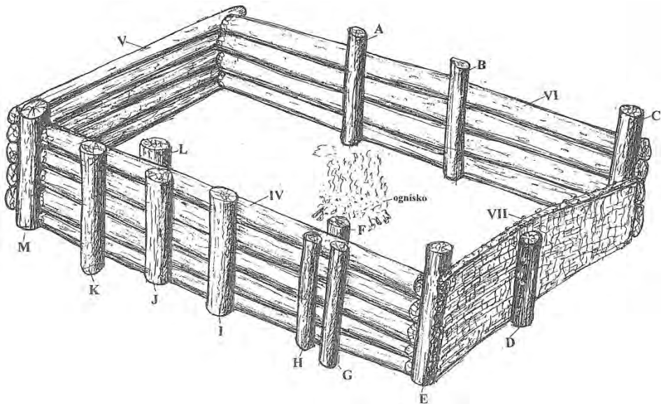
Ryc. 8. Broniszowice, pow. Ostrowiec Świętokrzyski, stan. V-A. Widok aksonometryczny zrekonstruowanego „domu kultowego” grobowca. A-M – słupy pionowe; I, II, III – belki rozporowe; IV, V, VI – ściany boczne; VII – wejście i plecionkowe drzwi (wg: Bąbel 2006, ryc. 11)
