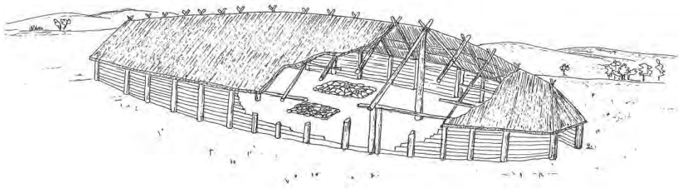
Ryc. 6. Pawłów, pow. Sandomierz, woj. świętokrzyskie, stan. 3. Rekonstrukcja budowli słupowej (sanktuarium) ludności kultury pucharów lejkowatych (wg: Bargiel, Florek 2002, s. 30)
