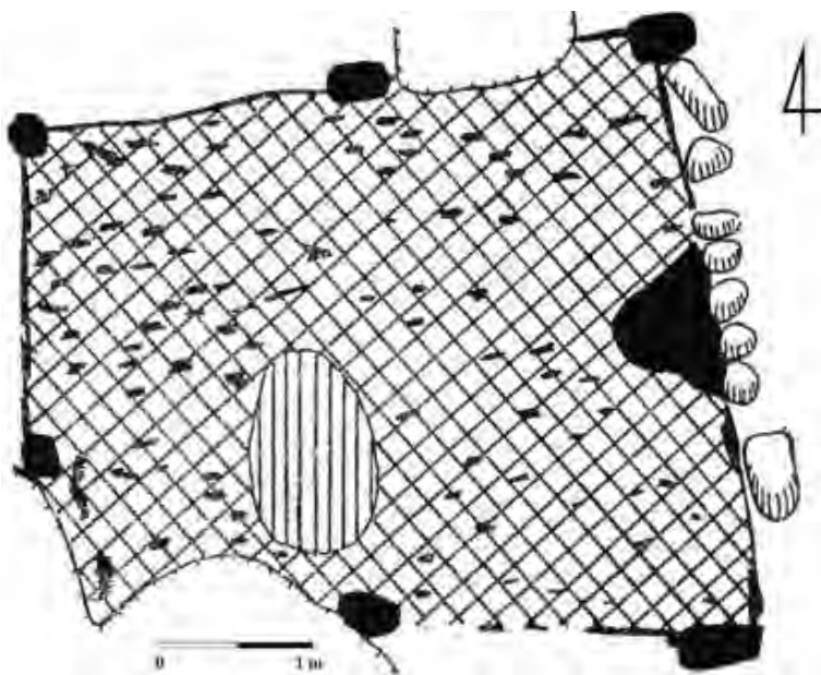
Ryc. 2. Gaj, pow. Koło, woj. wielkopolskie, stan. 1. Rzut poziomy „domu kultowego” (wg: Chmielewski 1952, ryc. 52)
