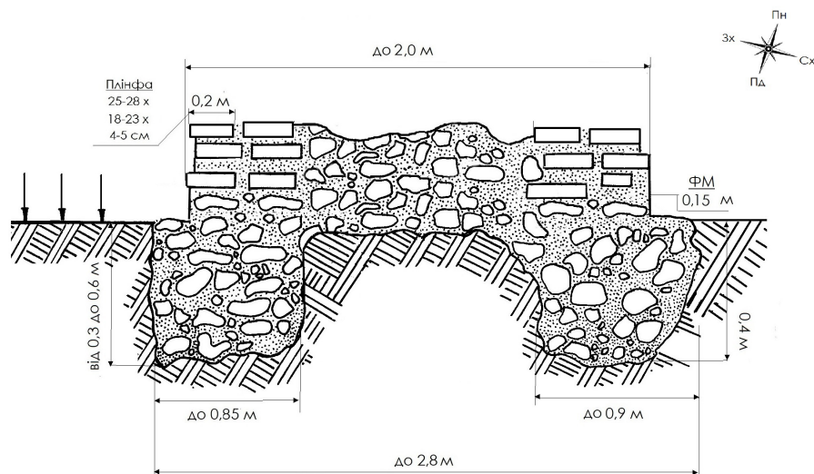
7. Реконструкція мурів XII ст. Печерського монастиря (автор С. Тараненко)
